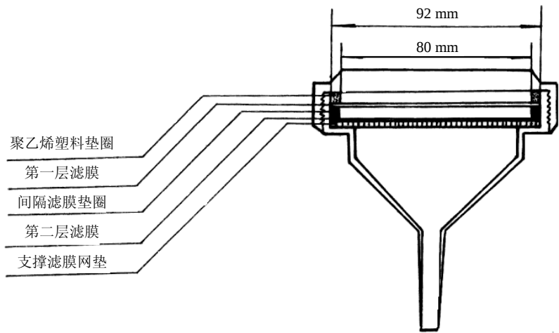
图 1 滤膜采样头装置
