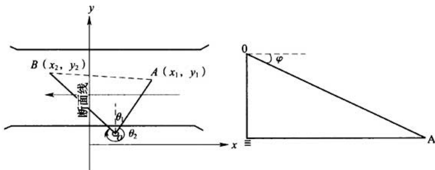
图 C. 7. 7-1 极坐标浮标法测流布置示意图
