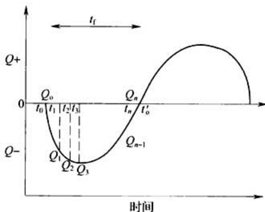
图 B. 7. 7 涨落潮潮量计算
