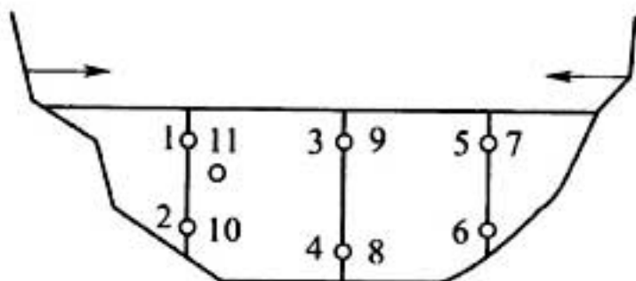
图 B. 3. 12 一船多线法试施测点次顺序
