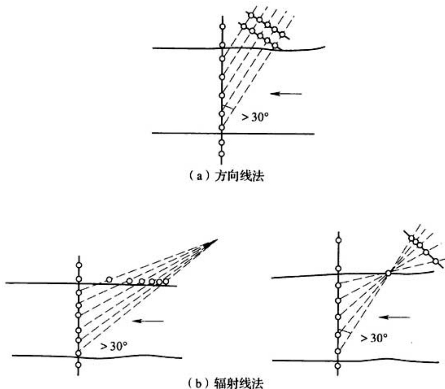
图 2.2.12 辐射线及方向线
