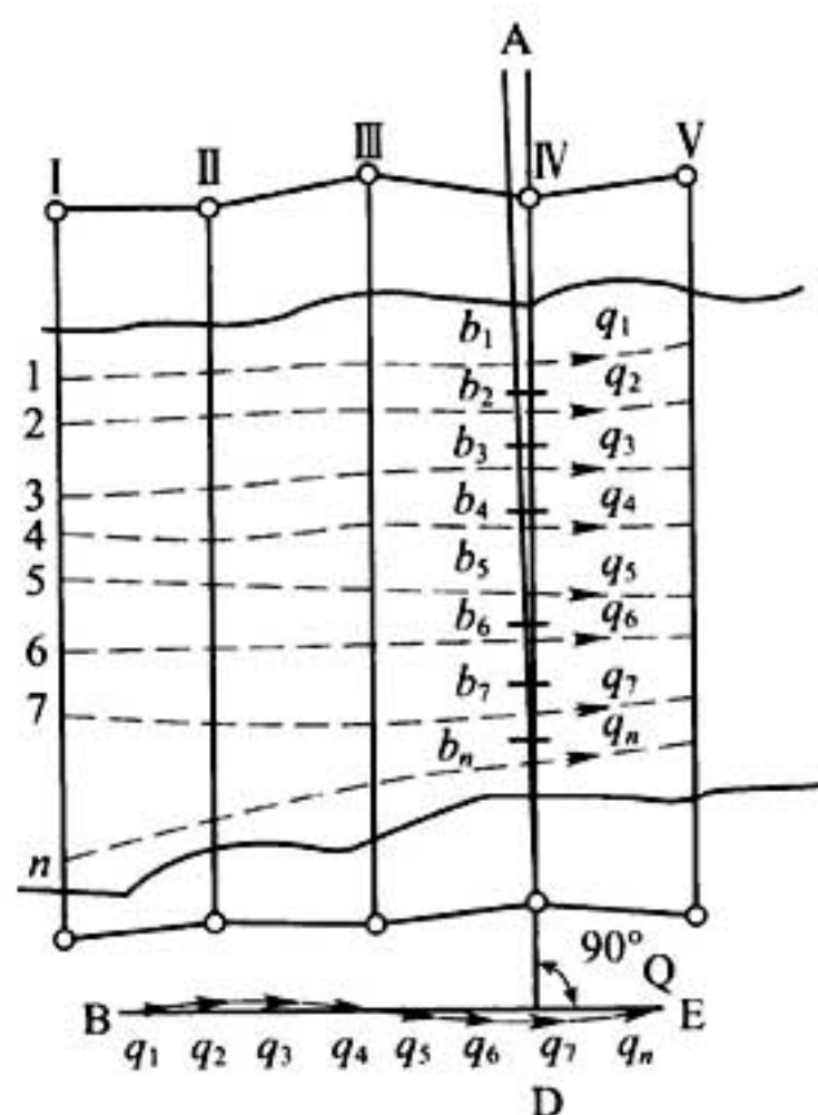
图 B. 10. 7 断面控制法
