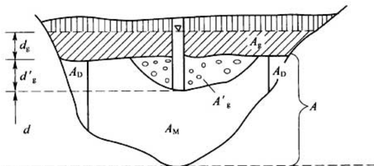
图 B. 7. 4 封冻期测流断面
