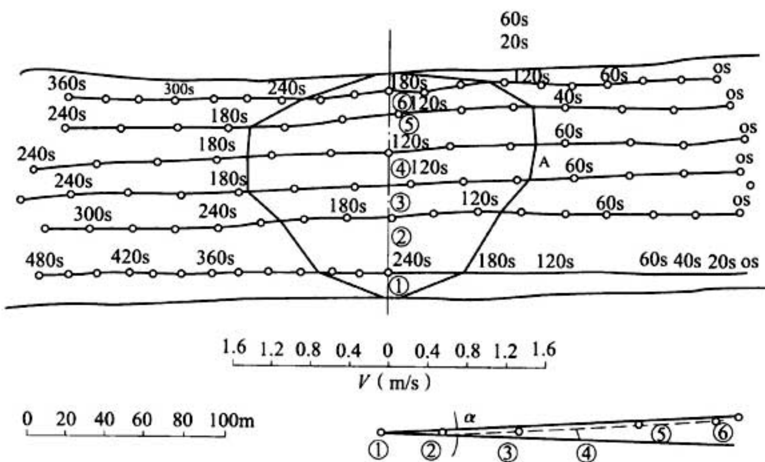
图 B. 10. 8 时间控制法
