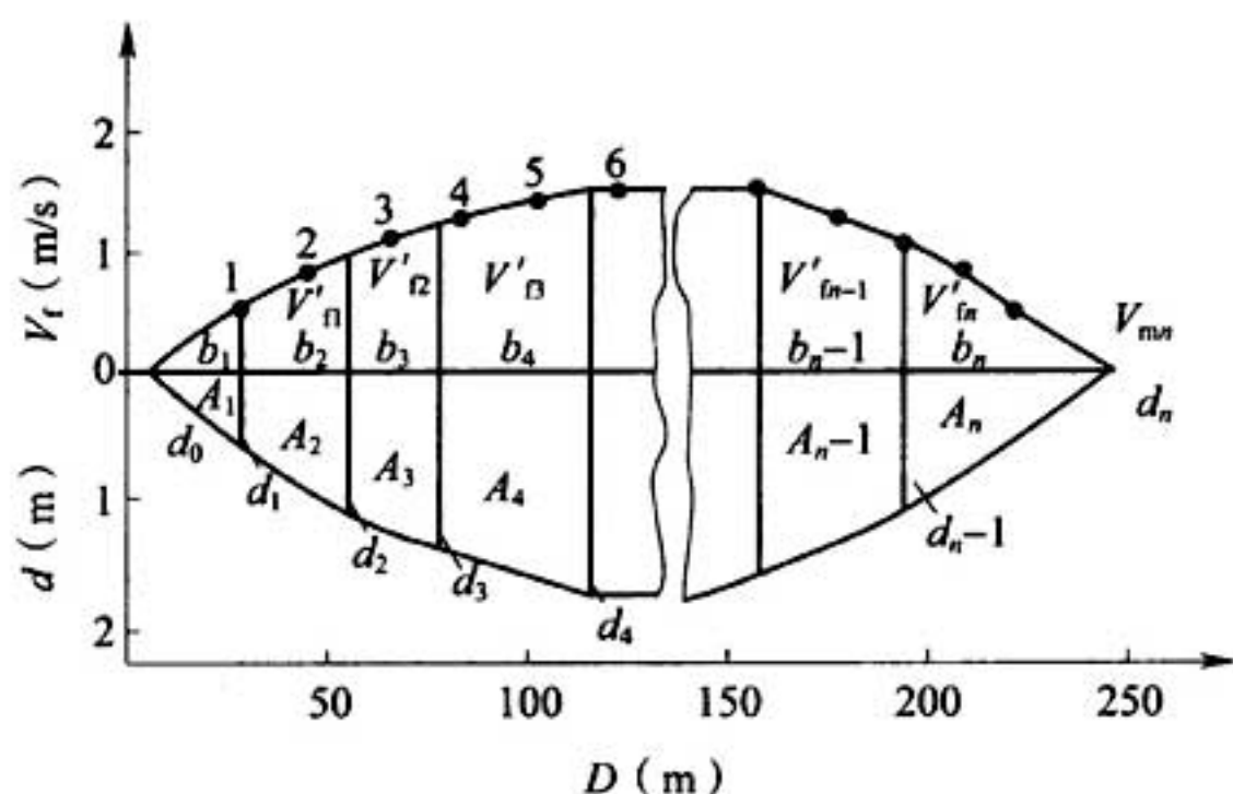
图 C.7.1 图解分析计算流量
