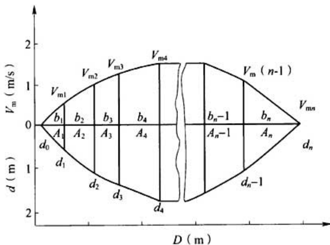
图 B. 7. 1 部分面积计算划分
