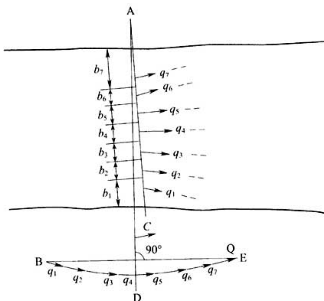
图 B. 10. 5 施测流速流向确定测流断面方向
