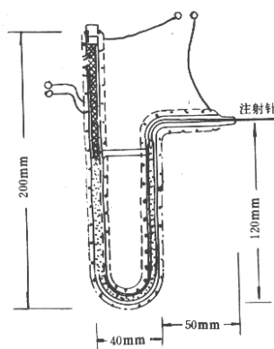
图 4 浓缩管
