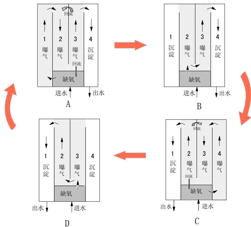
图 A.3 AICS 脱氮组合工艺流程
