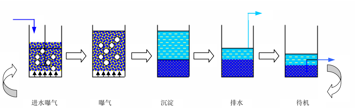
图 2 SBR 工艺运行方式——非限制曝气进水
