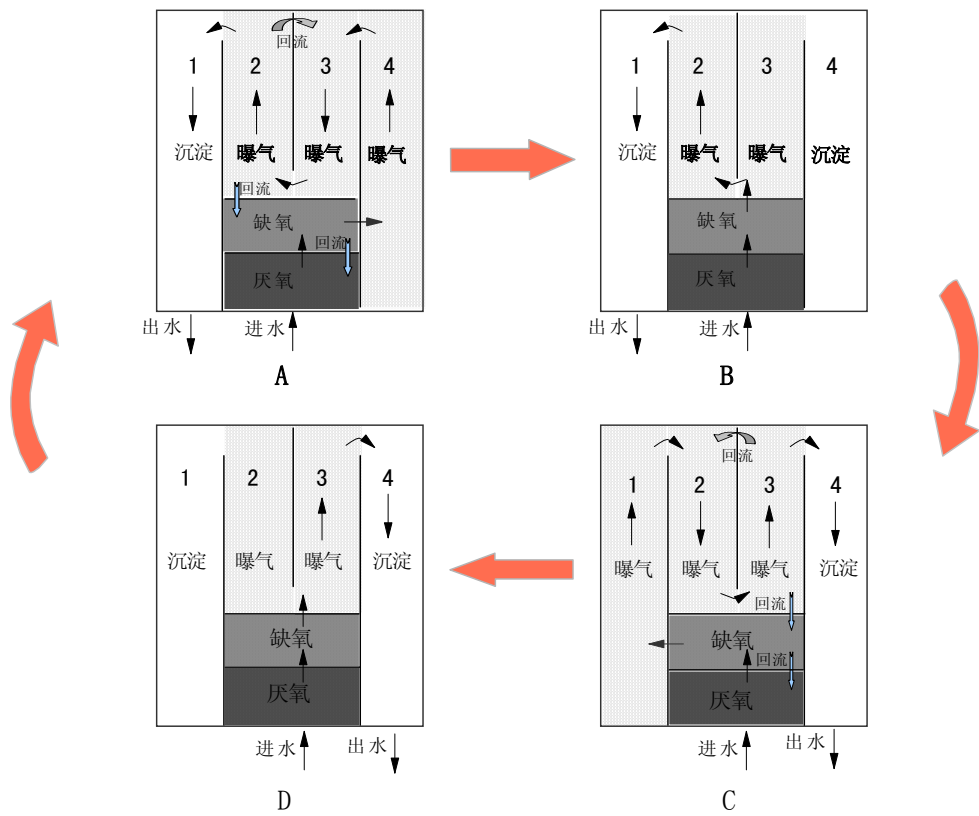
图 A.4 AICS 同步脱氮除磷组合工艺流程
