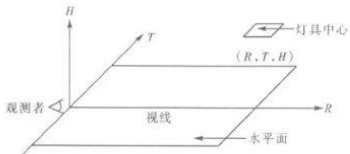
图 A.0.1 以观察者位置为原点的位置指数坐标系统 (R, T, H) ，对灯具中心生成 H/R 和 T/R 的比值
