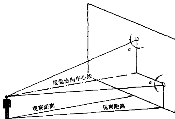
图 1 标志牌平面与视线夹角 \alpha 不低于 75^\circ
