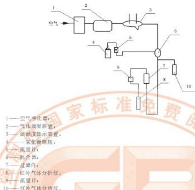
图 14 B 法动态气体吸附装置示意图
