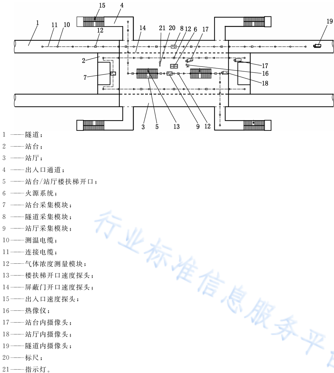
图 I.3 现场热烟测试设备布置方式示意图
