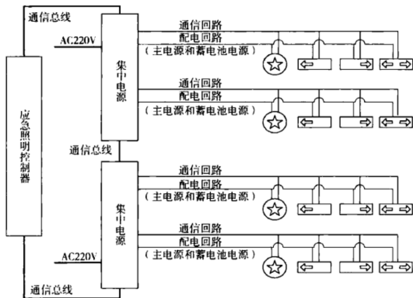
图 16 应急照明控制器与集中电源之间采用环形通信总线的集中控制型系统
