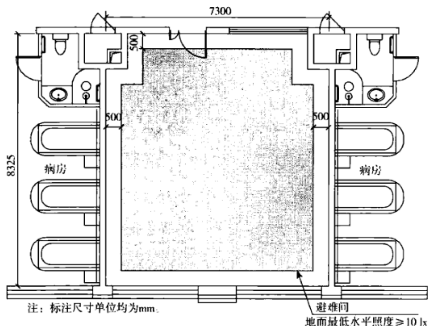
图6 病房楼的避难间地面水平最低照度
