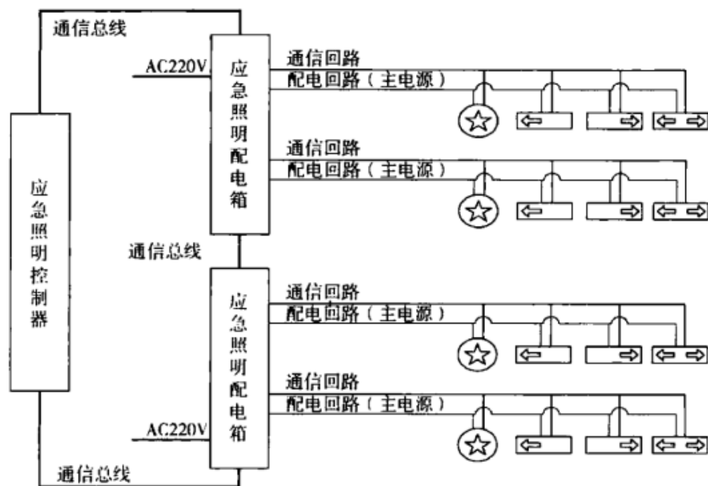
图 18 应急照明控制器与应急照明配电箱之间 采用环形通信总线的集中控制型系统
