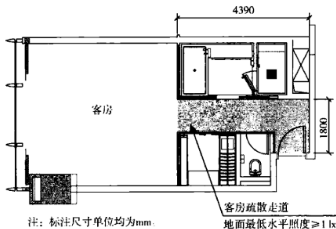
图 14 宾馆、酒店客房地面水平最低照度
