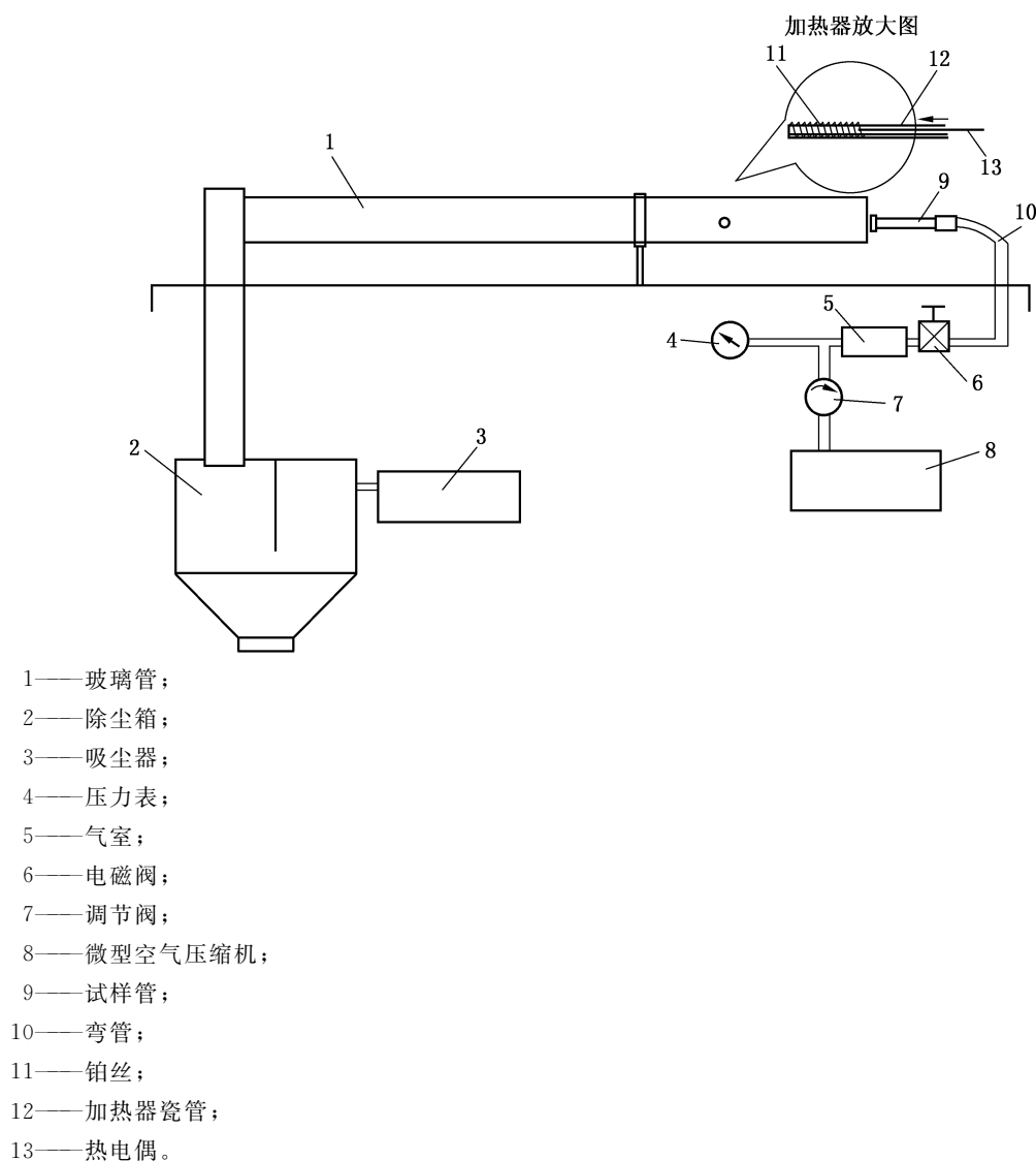
图 1 煤尘爆炸性鉴定装置示意图
