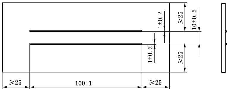
图 A.1 表面电阻测量试块
